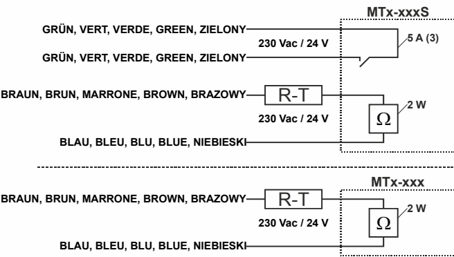
Fig. 4. Wiring diagrams
